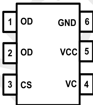
引脚示意图
