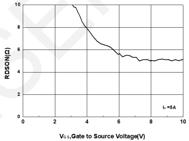
R_{DS(ON)} - V_{GS}
