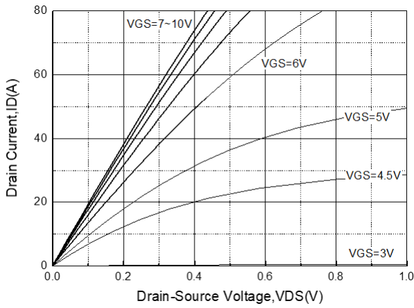
I_D - V_{DS}
