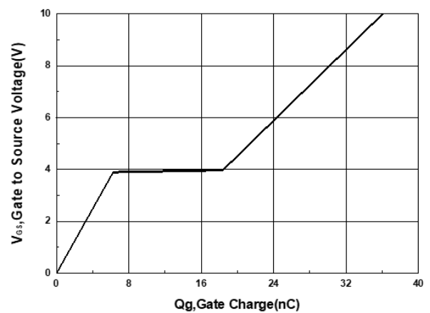
V_{GS} - Q_G
